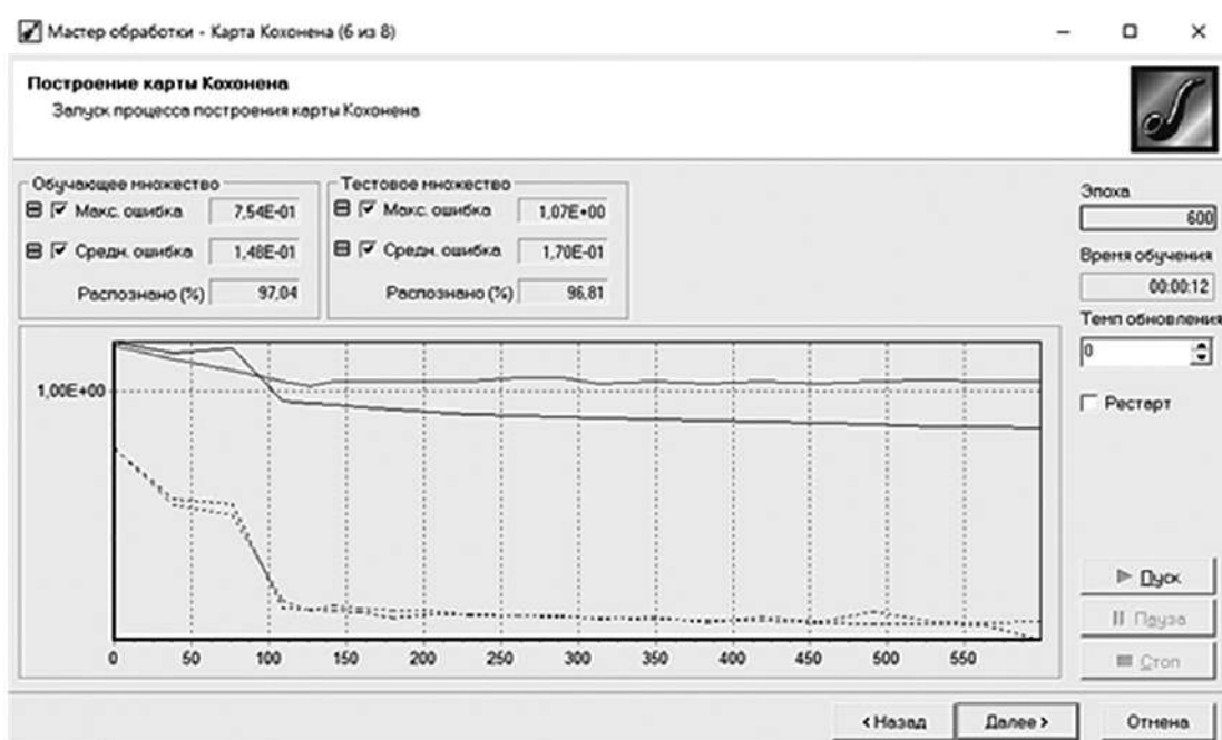
Рис. 5. График обучения
